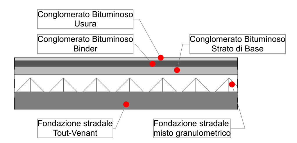
A-A PARTICOLARE SEZIONE STRADALE
