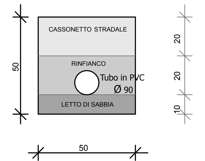
Part. B - CAVIDOTTO PUBBLICA ILLUMINAZIONE
