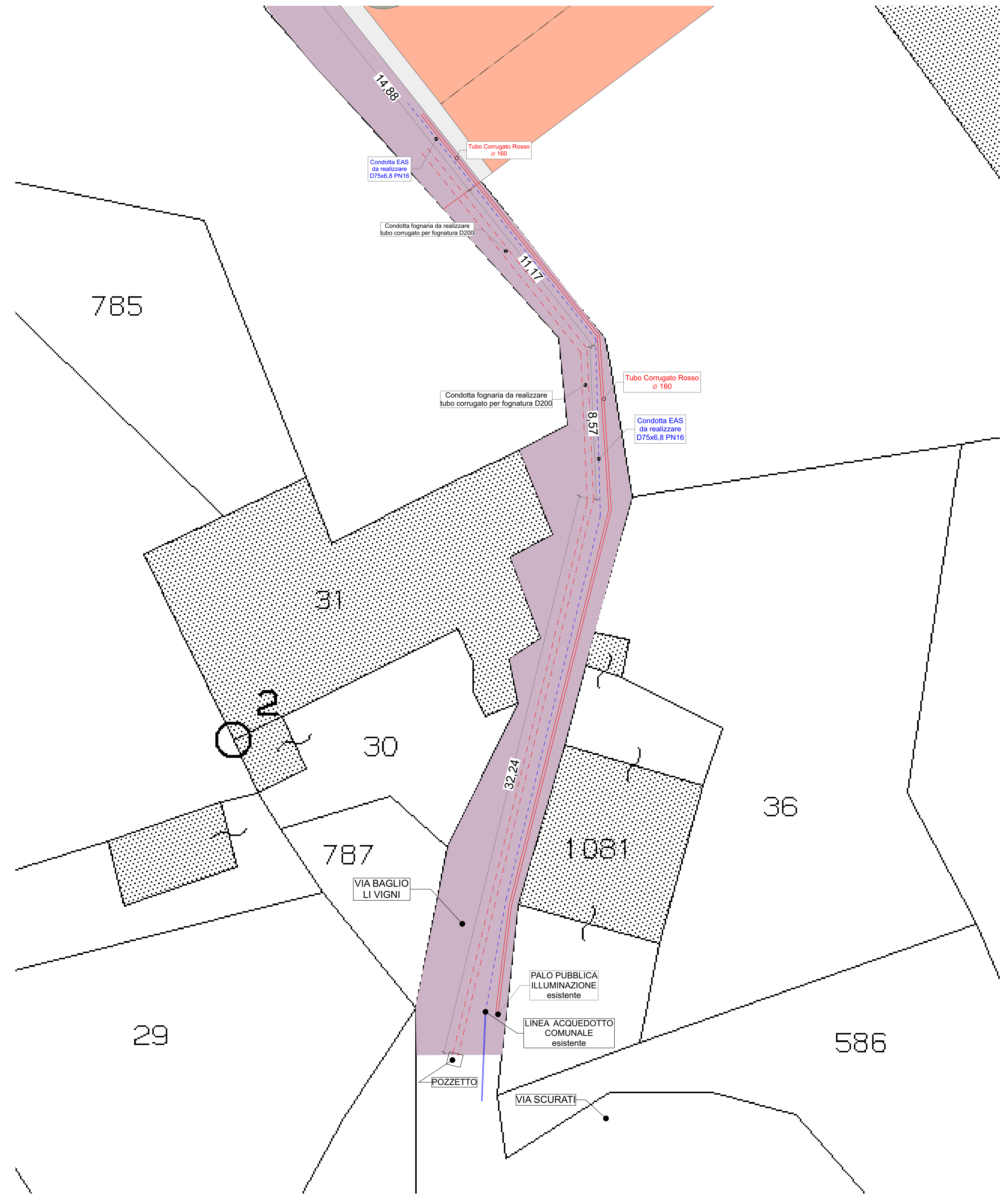
Part. B - CAVIDOTTO PUBBLICA ILLUMINAZIONE
